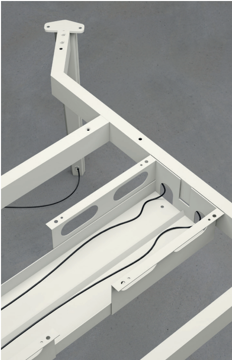
Doppia trave tavoli riunione P. 1200 Double beam meeting tables P. 1200
